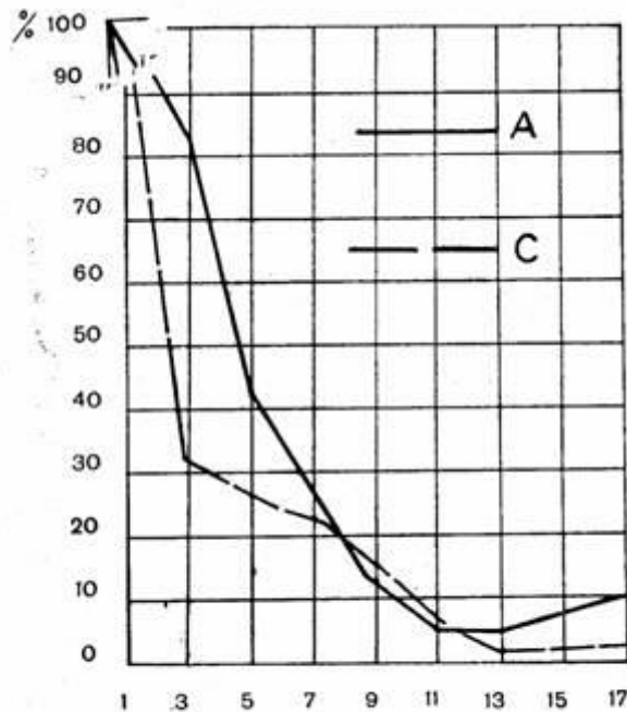
5-расм. Чистотириш эгри чизиклари: абсцисса — уринишлар сони; ордината—биринчи уринишга нисбатан процент ҳисобида ўлчанадиган вақт (масофа).
