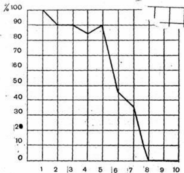
2-расм. Машқлар эгри чизиги: абсцисса— бир хил турдаги масалалар миқдори; ордината— хатоларнинг бошланғичга нисбатан процент ҳисобидаги миқдори.
