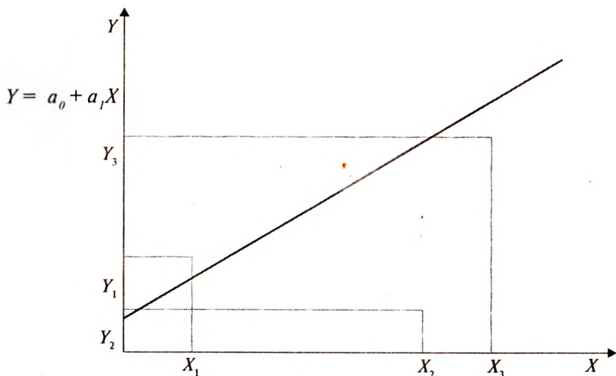
11- чизма. Чизиқли бир омили боғлиқлик графиги.
