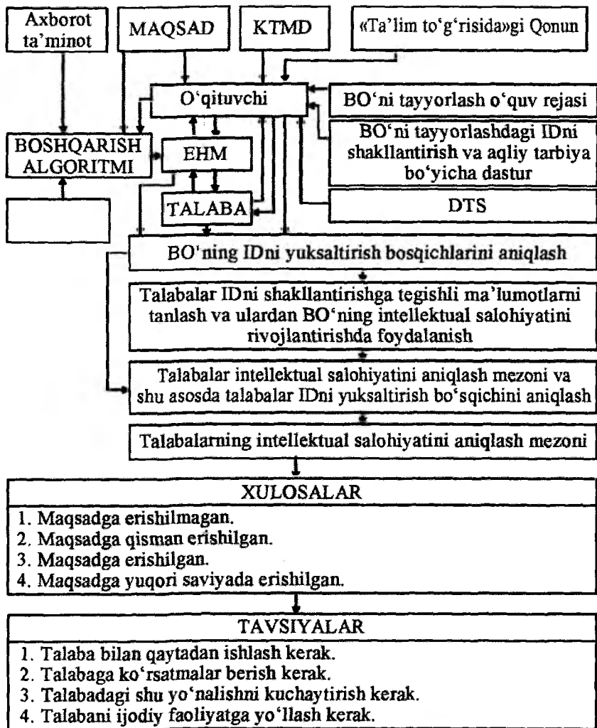
9.1.1-shakl. Ko'makchi kompyuterli tizim ishlashini tashkiliy-tuzilmaviy modeli.
